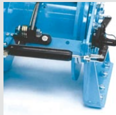
Pneumatische Kupplungsbetätigung für erhöhten Bedienkomfort
